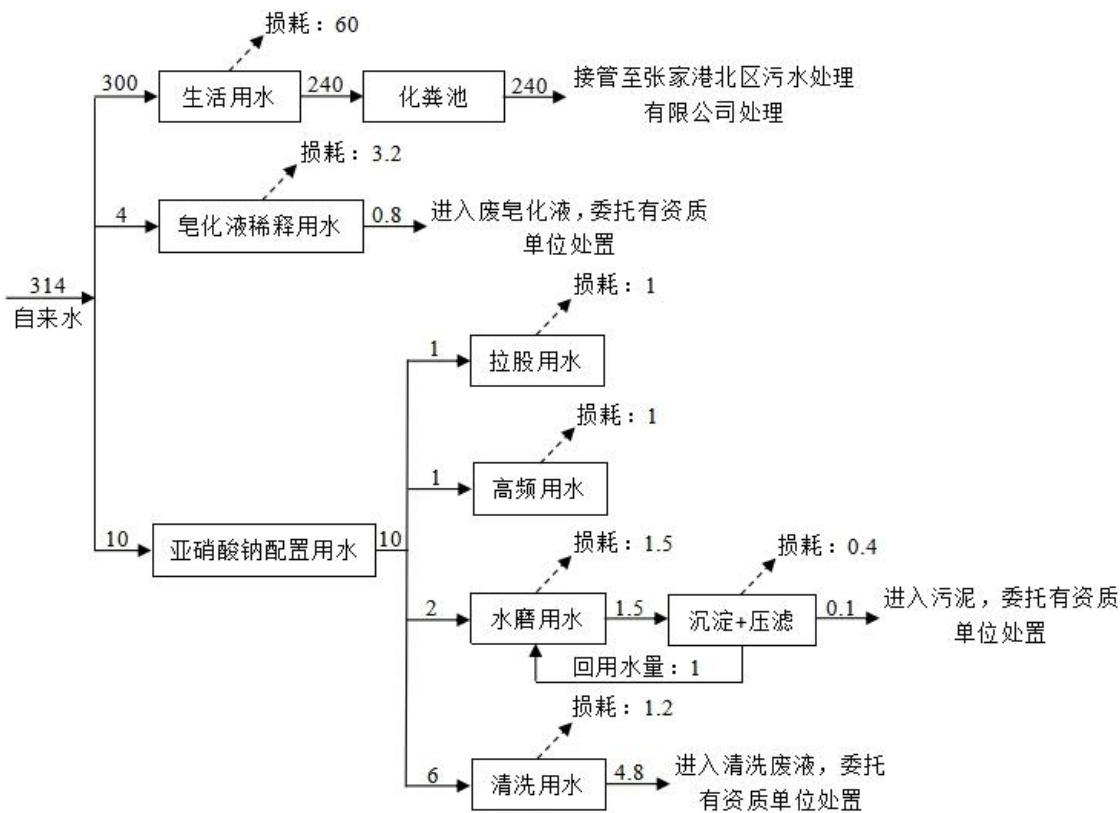
图 2-1 本项目水量平衡图 单位：t/a
