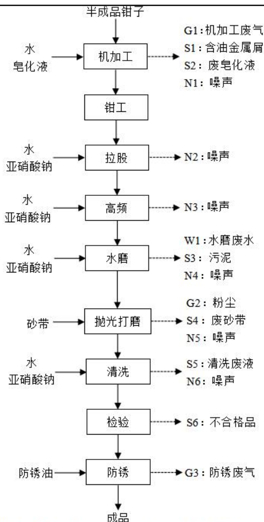
图 2-2 本项目生产工艺及产污环节流程图
